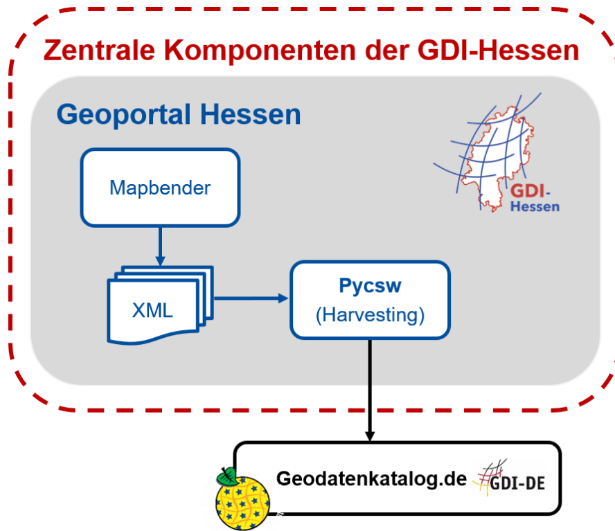
Abbildung 7 - Anbindung der GDI-Hessen an den Geodatenkatalog.de
