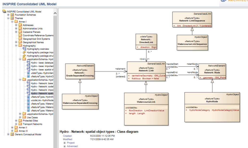
Abbildung 21 - UML-Diagramm
